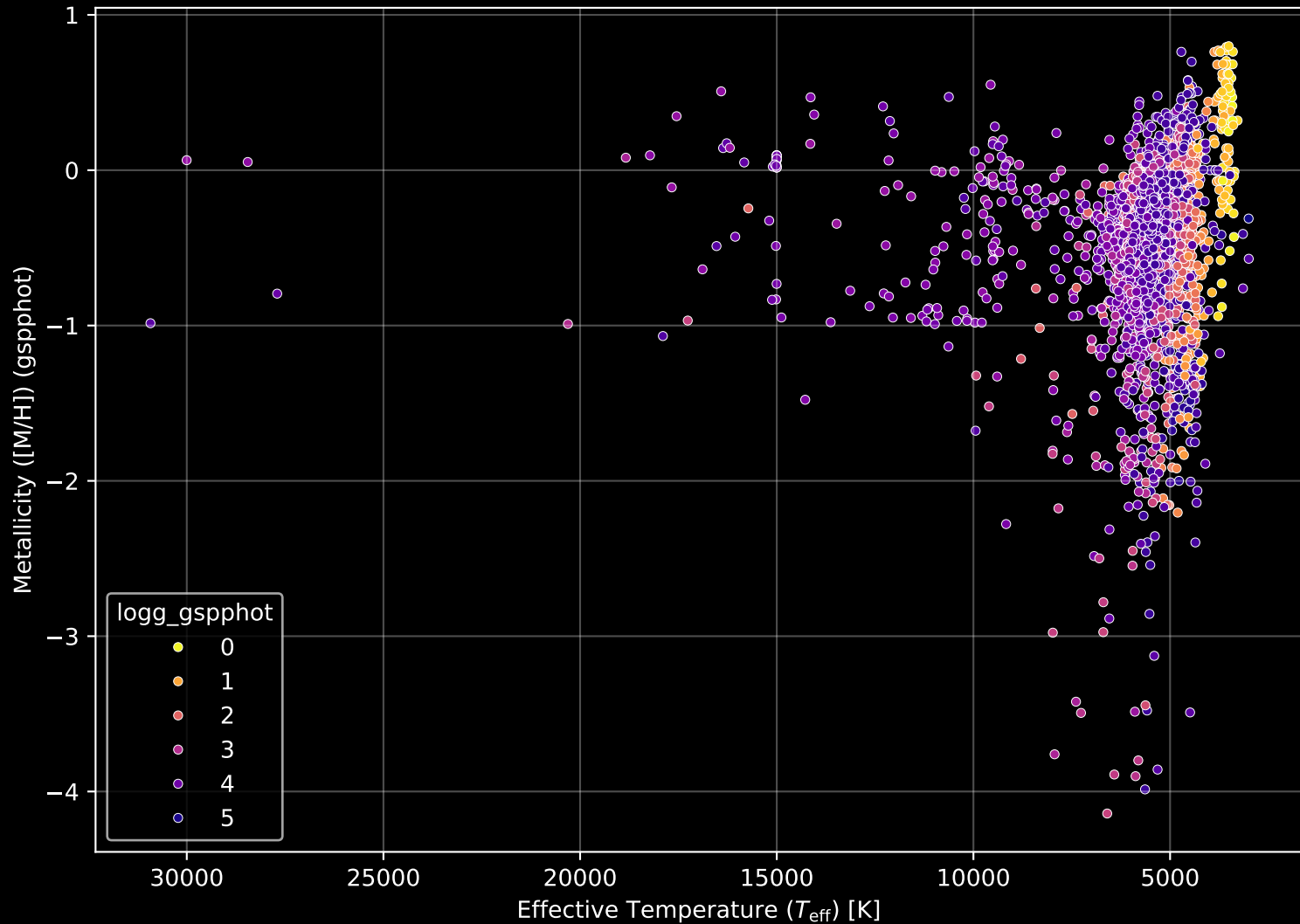
GALAH DR4 Field: [-6] Stellar Population Parameters (n= 3442)
