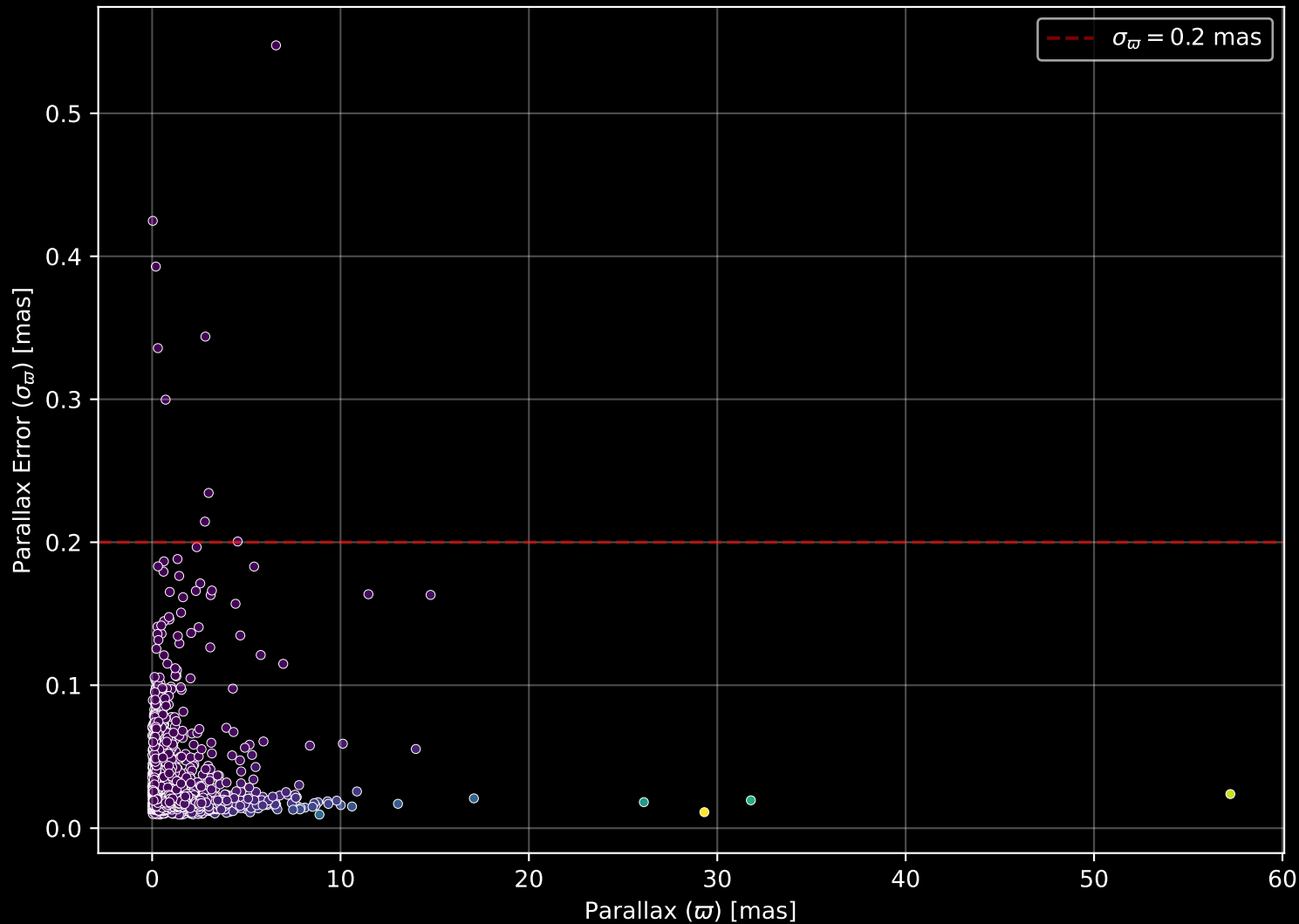
GALAH DR4 Field: [-6] Parallax Quality (n= 3442)
