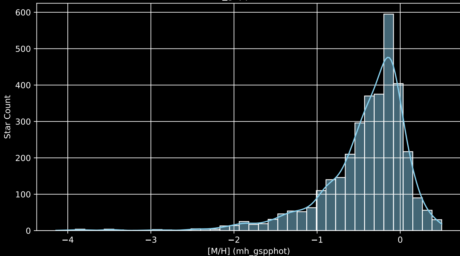
GALAH DR4 Field: [-6] [M/H] (mh_gspphot) (n= 3407)
